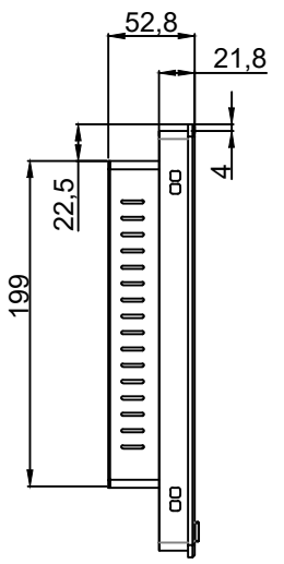
前置USB15.6寸外嵌式（散热款）
